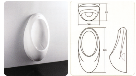
NEW [Urinal] ▶ C U-900 (물안쓰는 소변기)
